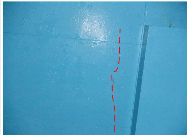
배수지2지 상부슬래브 균열
