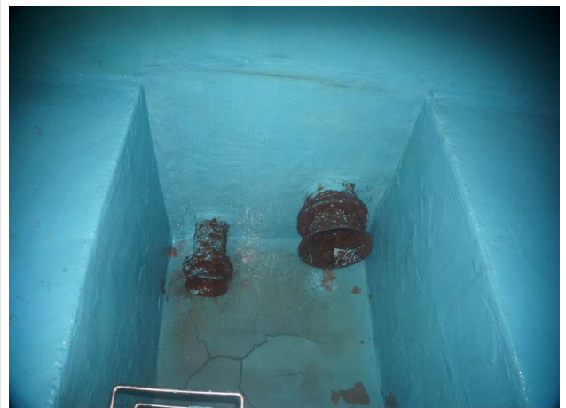
1지 배수지 유출배관 관부식
